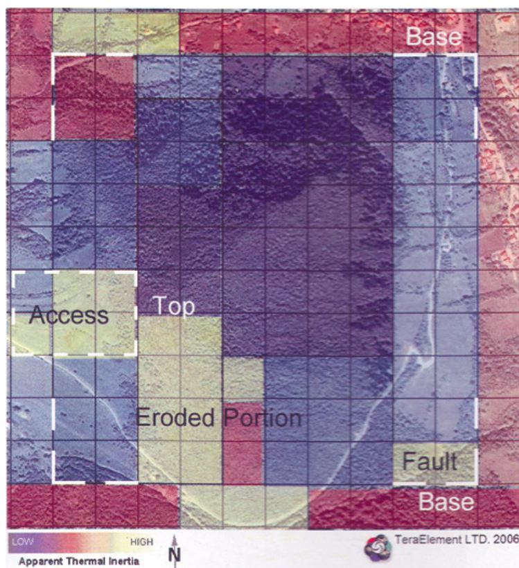
Satelitska toplotna karta, snimljena s instrumentom Aster na satelitu Terra koji je u zemaljskoj orbiti od 1999. godine, po objašnjenju dr. Amera Smailbegovića, pokazuje da se te uzvisine, piramide, hlade brže od ostalih, jer su iz drugog, manje gustog odnosno više poroznog kamena, što znači da su šuplje. Na slici su tamnija polja tamo gdje je piramida Sunca.
